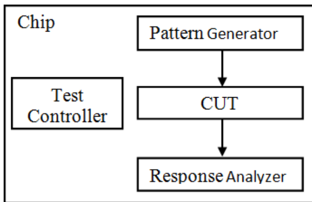
Fig. 1: A Generic BIST Module
